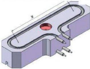
Man6-Y Manifold Rezistansı
