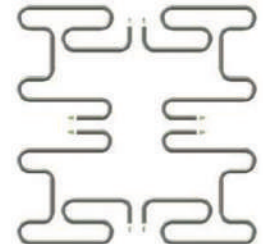
Man16-4H Manifold Rezistansı
