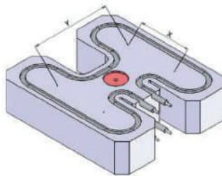
H TİPİ 4 ENJEKSİYONLU
